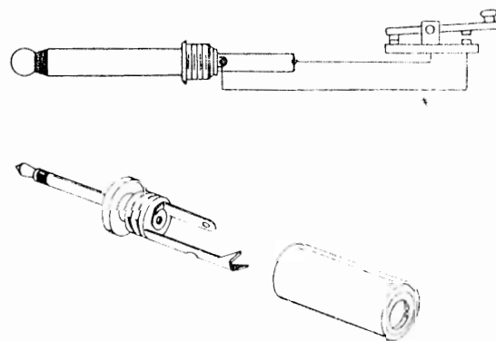
第3図 キープラグの接続
