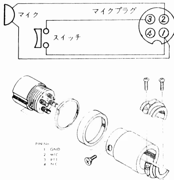
第1図 マイックプラグの接続
