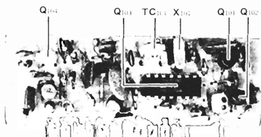
RF/MARK UNIT (PB-1884)
