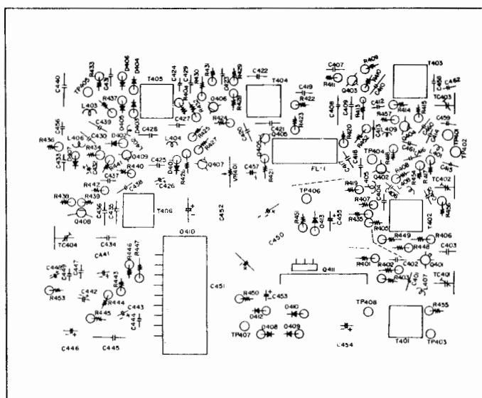
IF-AF UNIT(PB-1528)
