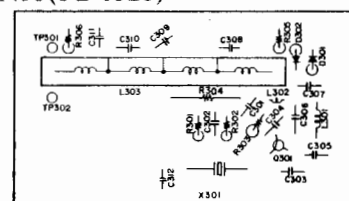
HG UNIT(PB-1524)
