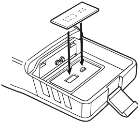
気圧センサーユニットをコネクタに差し込み、付属のシールを貼った後、電池パックを取り付けます。
