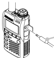
EAR 端子に市販のステレオイヤホンを接続する
