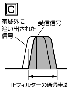
IFフィルターの通過帯域幅
