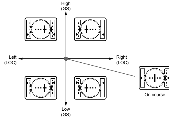
Ejemplos de CDI correspondientes a la ubicación de los aviones (La pista tiene que estar en la parte trasera de la pantalla)
