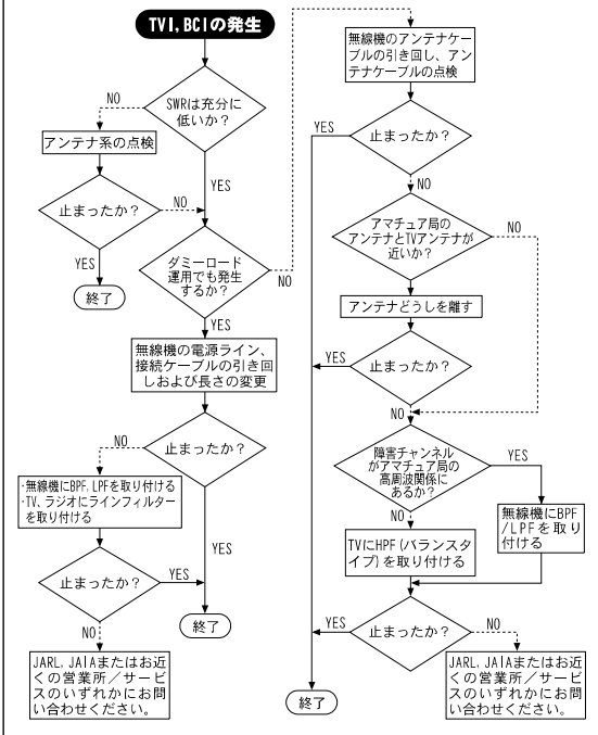
電波障害(TVI, BCI)対策フローチャート (例)
