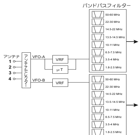
\mu -TUNE/VRF回路 概念図
