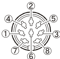
BAND DATA に接続するプラグ結線図
