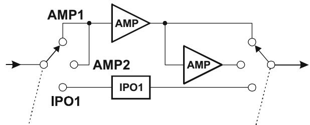
VFO-B 受信 RF アンプ部
