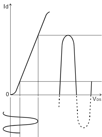
AB級動作
