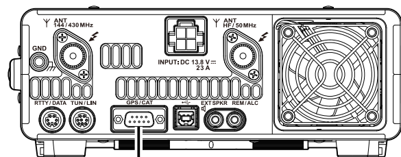
[GPS/CAT]端子
