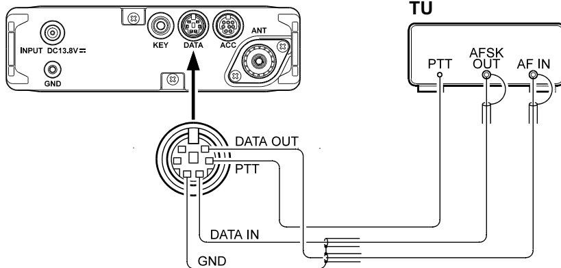
パケットケーブル CT-39A (オプション)
