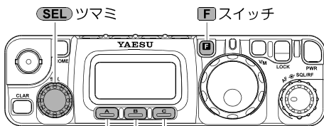
マルチファンクションキー
