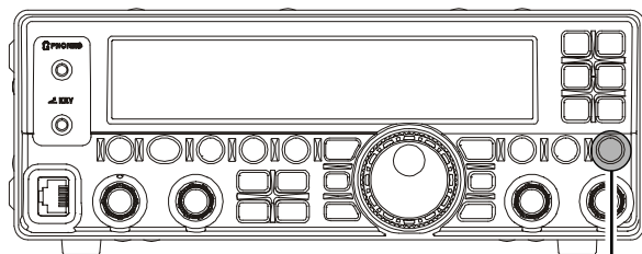
[ METER/DIM ]スイッチ
