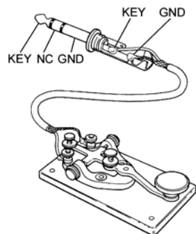
縦振れ電鍵の接続
