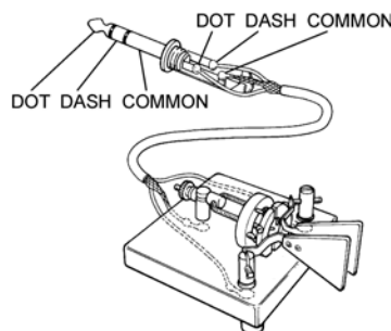
パドルの接続
