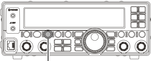
[ATT/IPO]スイッチ
