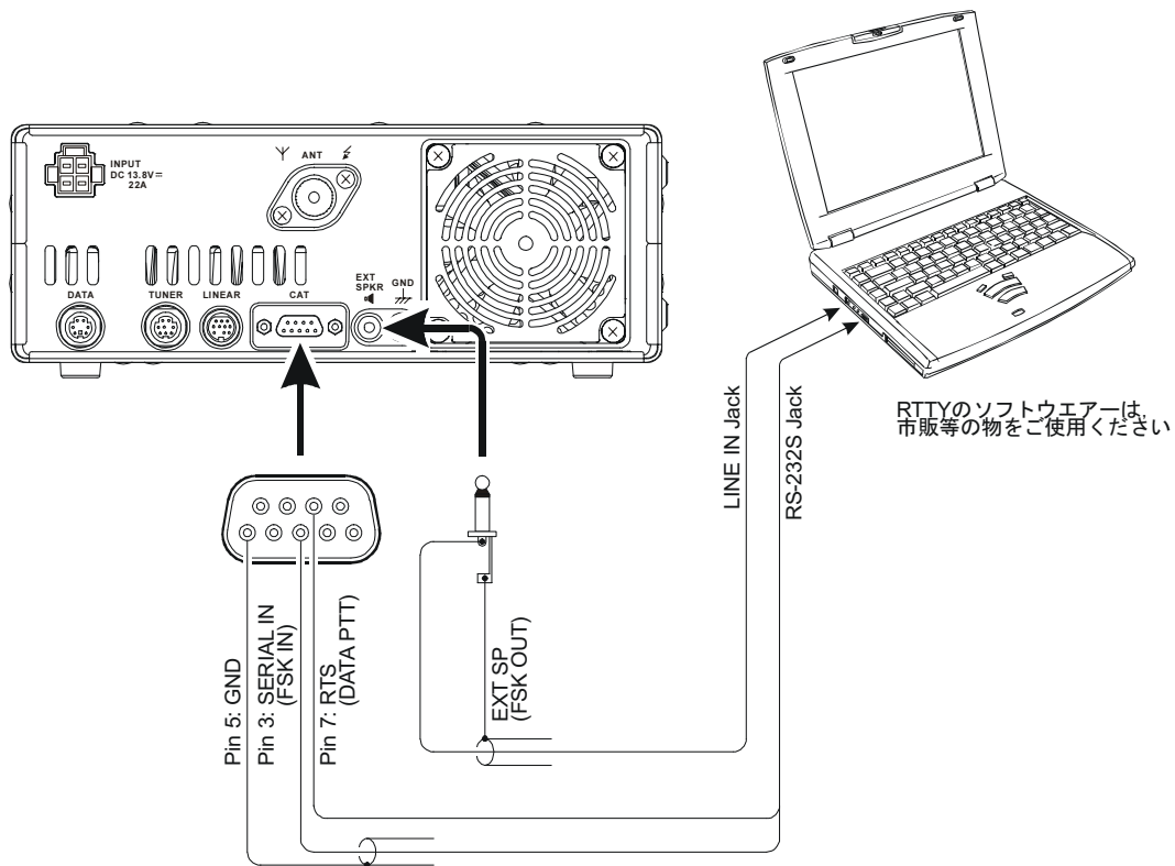
「CAT RATE」の “DATA” による接続例
