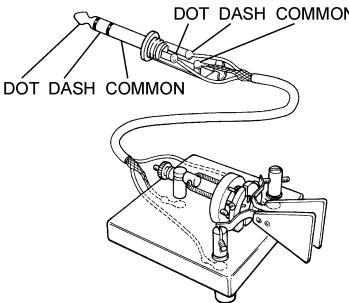
パドルの接続
