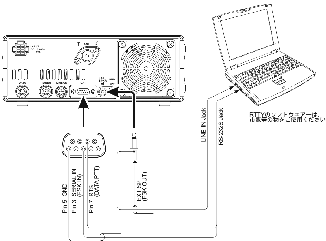
「CAT RATE」の “DATA” による接続例
