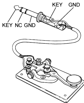
縦振れ電鍵の接続
