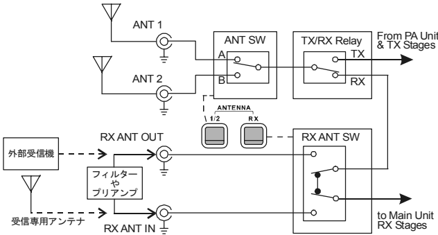
アンテナ回路構成
