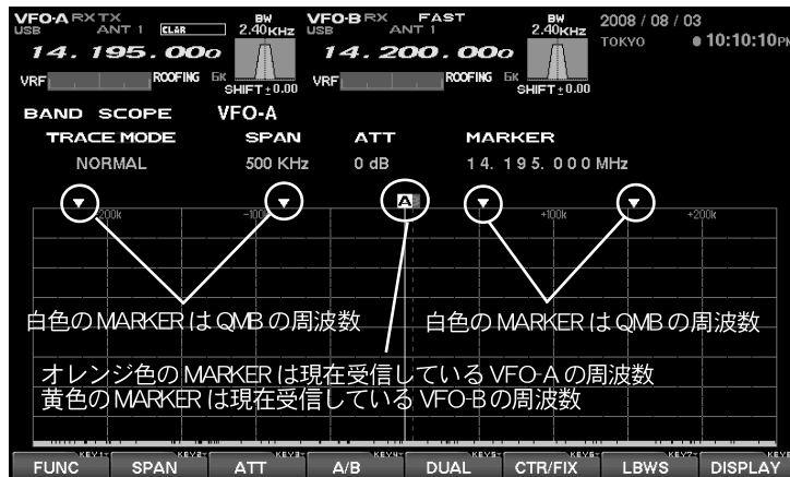
上図は 14MHz 帯に 4 チャンネルの QMB MARKER を表示されている例
