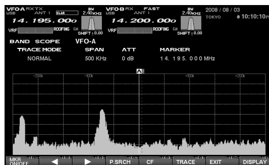
↑ マーカー設定画面
