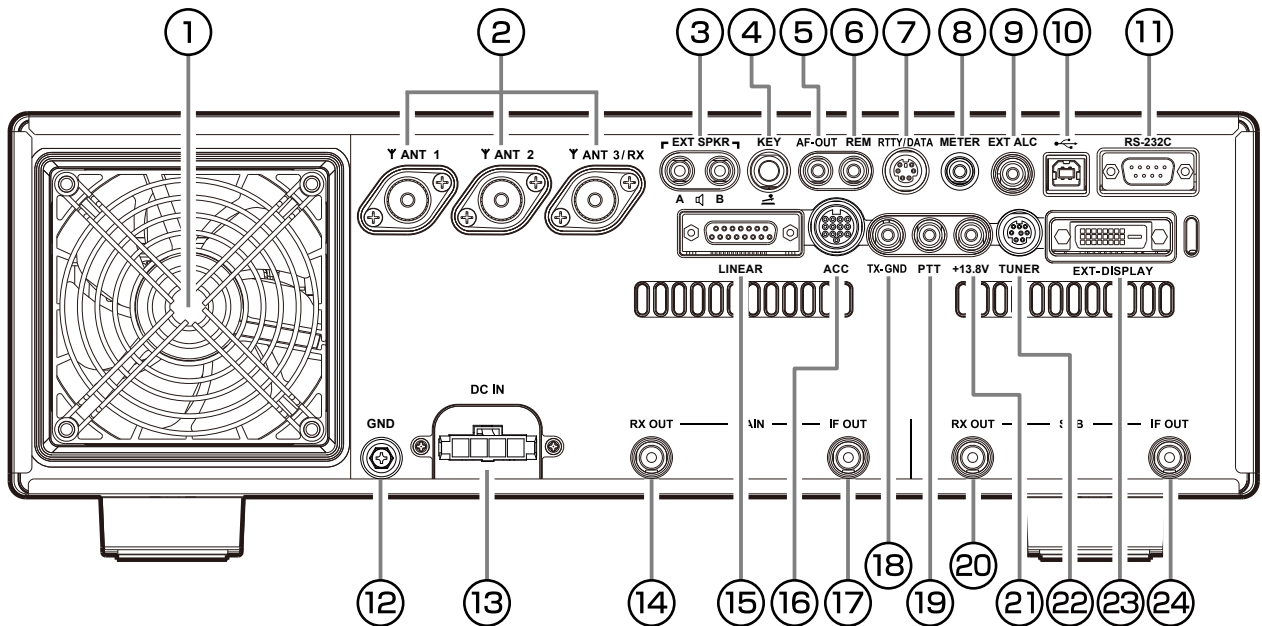
La figure ci-dessus représente le panneau arrière du FTDX101MP.
