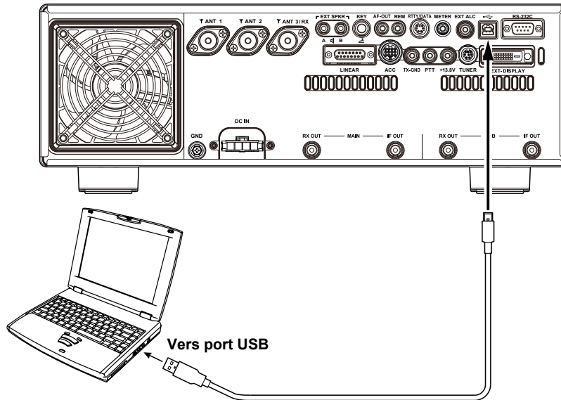
Câble USB (A-B) disponible dans le commerce
