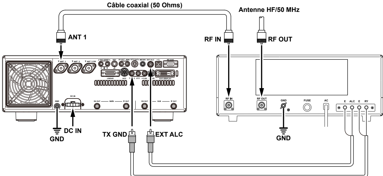
La figure ci-dessus représente les branchements du panneau arrière du FTDX101MP à d'autres amplificateurs linéaires.
