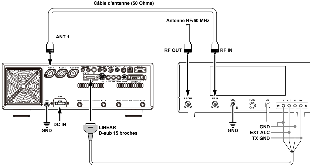
La figure ci-dessus représente les branchements du panneau arrière du FTDX101MP à d'autres amplificateurs linéaires.
