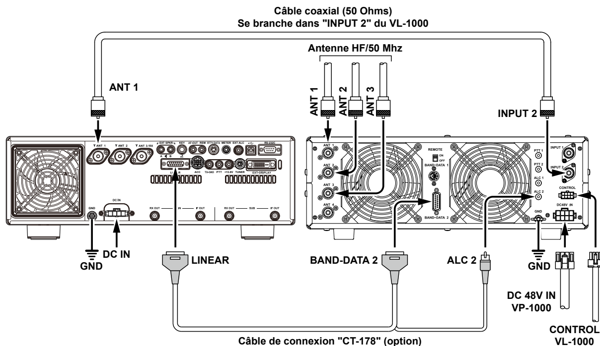
La figure ci-dessus représente les branchements du panneau arrière du FTDX101MP avec le VL-1000.
