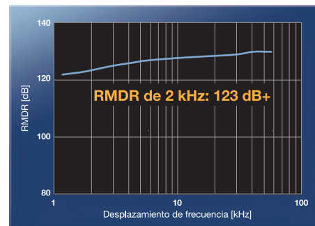
Mezcla recíproca en la banda de 14 MHz Rango dinámico (RMDR)
