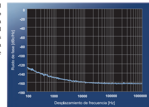
Unidad 400 MHz HRDDS
