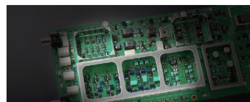
15 filtros pasa banda separados
