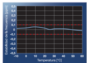
TCXO de alta precisión de \pm 0,1 ppm
