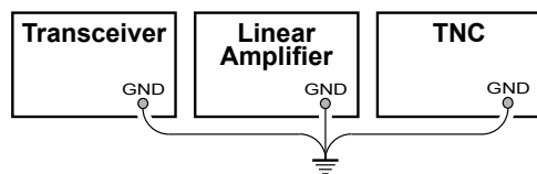
RICHTIGER ERDUNGSANSCHLUSS
