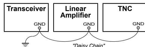
FALSCHER ERDUNGSANSCHLUSS
